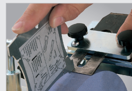
Winkellehre für Stein Ø 250 mm (Art.-Nr.: 5760052)
