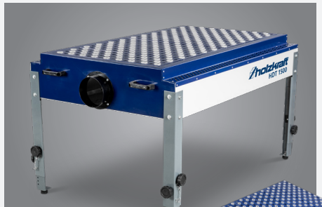
Metallauflegerost mit Gummiauflagen L x B: 1.350 x 693 mm
