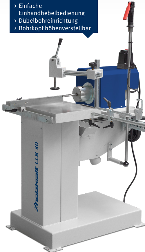
LLB 30 mit optionalen Winkelschlag
