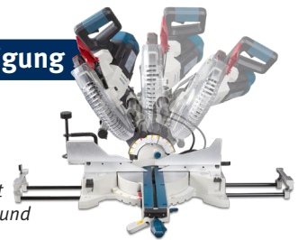
Ausziehbare Anlageschienen und ausziehbarer Tisch
