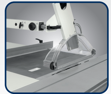
Sägeblattpendelschutz mit Absaughaube (manuell einstellbar)
