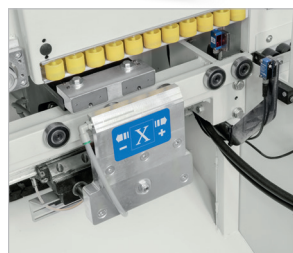
Pneumatische Spannzange für Werkstückpositionierung
