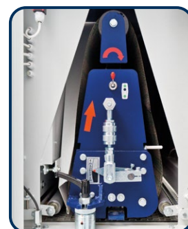
Serienmäßig mit gerippter Stahlwalze Ø 120 mm und hartem Schleifschuh mit Graphitbelag
