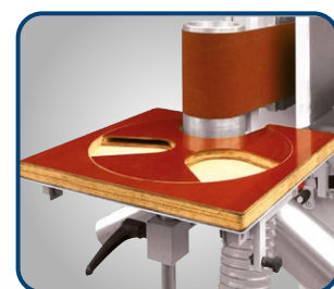
KSO 150 FD mit Drehstern und drehbarer Absaugplatte zum schnellen Umrüsten von 3 verschiedenen Schleifradien: Ø 60 mm, Ø 100 mm, Ø 120 mm
