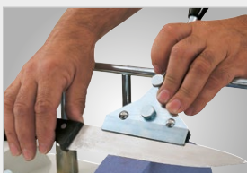
Vorrichtung für große Messer (Art.-Nr.: 5760057)
