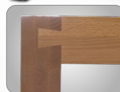
Schwalbenschwanzverzinkung in Hinterzange und Beiladerücken
