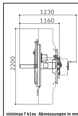
minimax f 41es Abmessungen in mm
