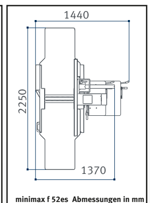
minimax f 52es Abmessungen in mm
