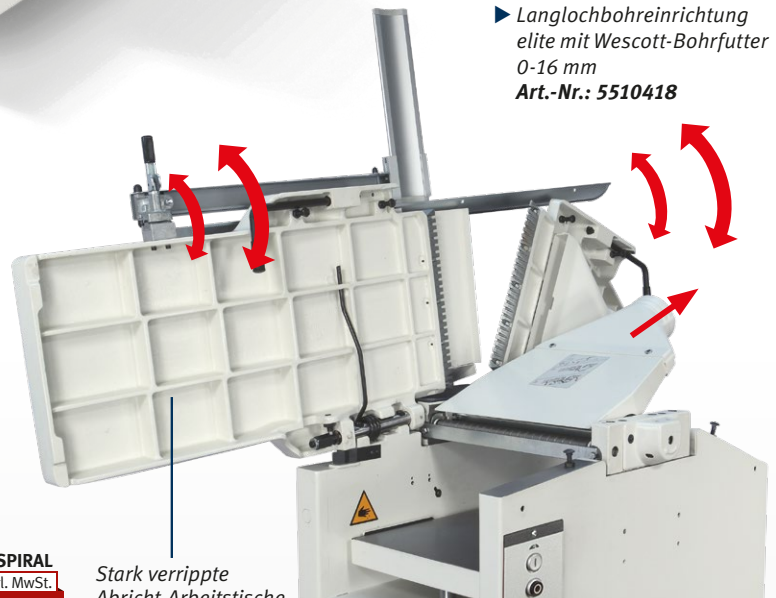
minimax fs 41e mit geöffneten Abrichttischen
