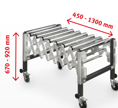
SRB 130 Scherenrollenbahn Höhe einstellbar, Rollenlänge 480 mm
