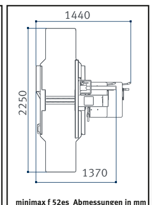
minimax f 52es Abmessungen in mm
