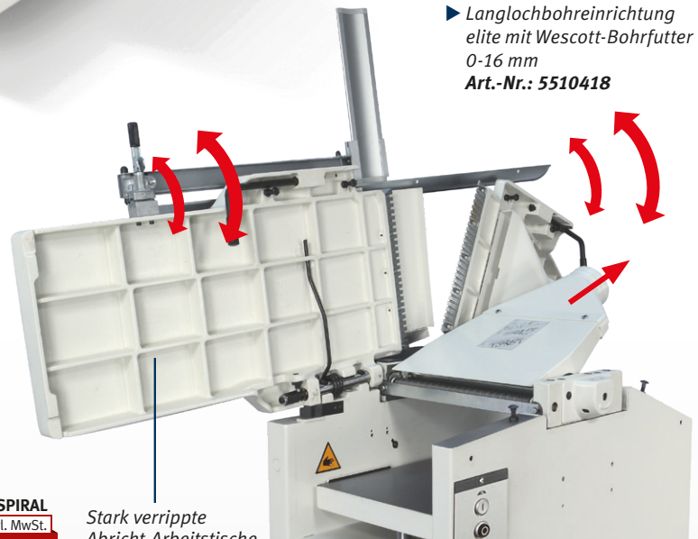
minimax fs 41e mit geöffneten Abrichttischen
