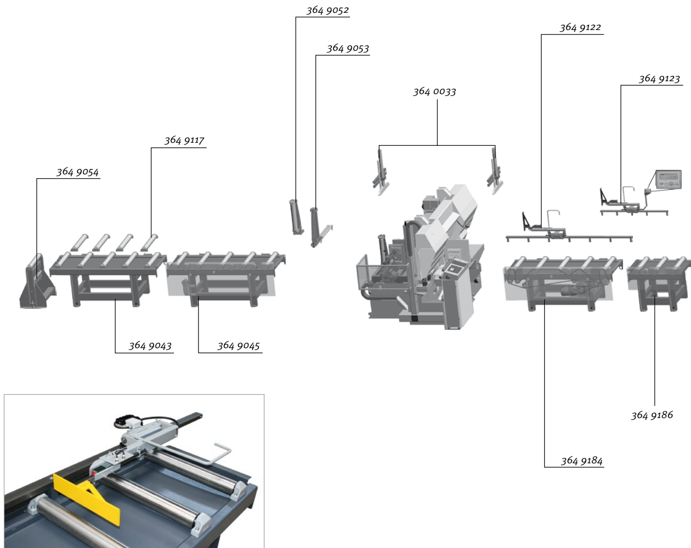
Abb.: Rollenbahn 600 mm mit Anschlag elektromechanisch
