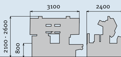
Abmessungen HMBS 510 x 510 CNC-FX
