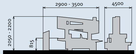
Abmessungen HMBS 450 x 600 NC-DG-FX 2000
