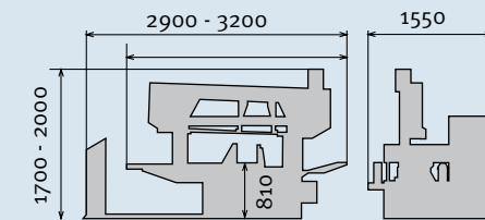
Abmessungen HMBS 350 x 500 HA-DG-FX
