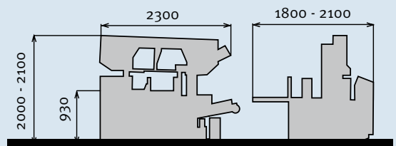
Abmessungen HMBS 350 x 400 CNC-F / CNC-FX
