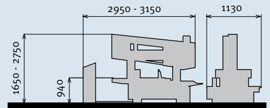
Abmessungen BMBS 460 x 600 HA-DG-F
