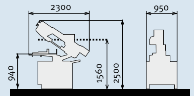
Abmessung BMBS 350 x 400 HA-DG-F
