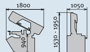
Abmessung BMBS 240 x 280 HA-DG / HA-DG-F
